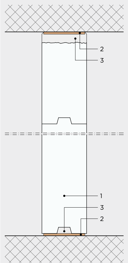
Sezione verticale
