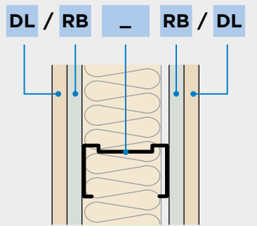
Esempio: parete a telaio, rivestimento a due strati, ibrido
