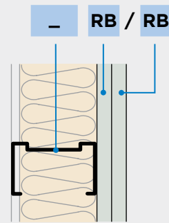
Esempio: controparete, rivestimento a due strati
